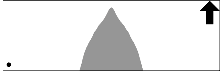
Laurier-tin
